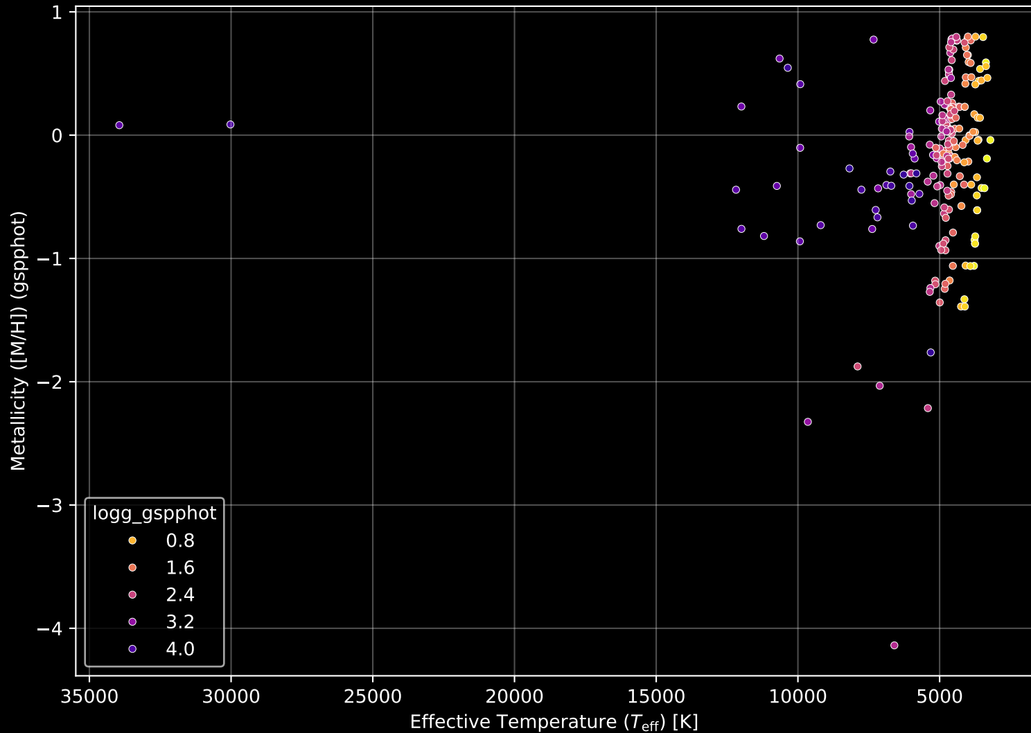
APOGEE DR17 Field: [006+02] Stellar Population Parameters (n= 215)
